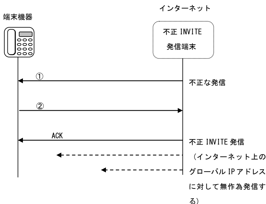
図 1.1 不正 INVITE リクエストに対する対応シーケンス
